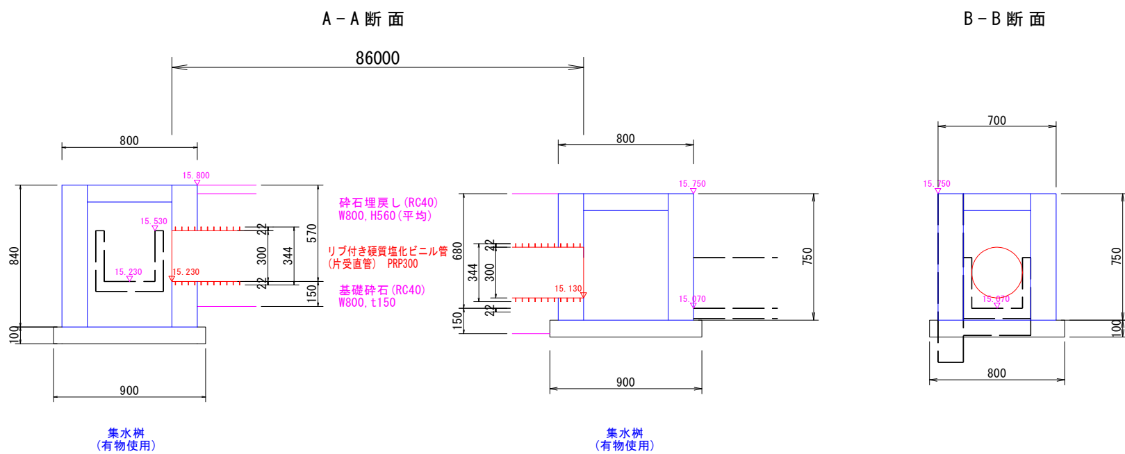
断面図
